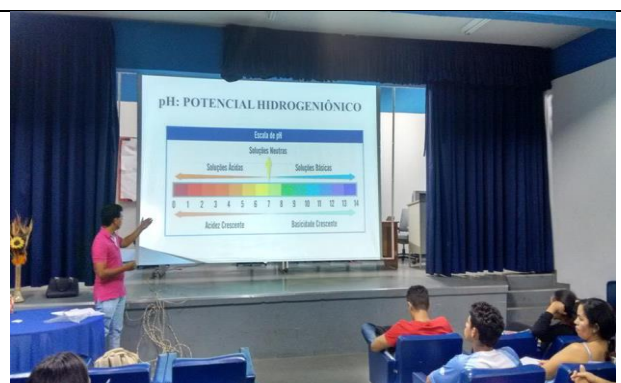
Escala pH (Potencial Hidrogeniônico) Distinguir Acidez e Basicidade
